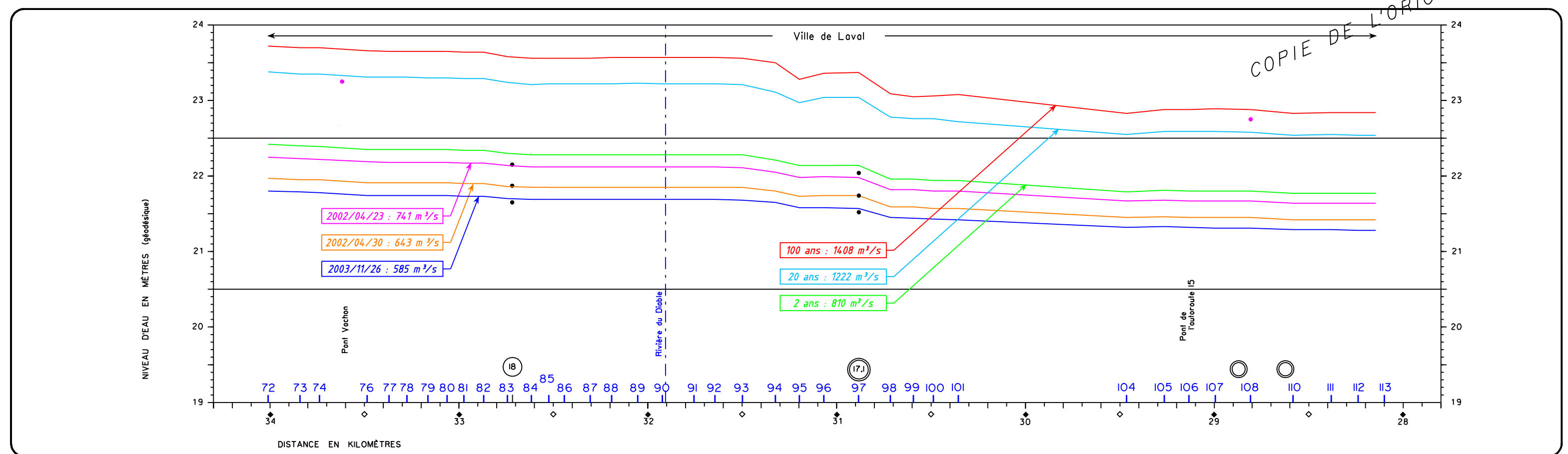
FIGURE 8 PROFIL DES PLANS D'EAU DE LA RIVIÈRE DES MILLE ÎLES SECTEUR DE BOISBRIAND LÉGENDE : Profil du plan d'eau de récurrence de 100 ans Profil du plan d'eau de récurrence de 20 ans Profil du plan d'eau de récurrence de 2 ans Site de calcul de niveaux d'eau Niveau d'eau observé Niveau établi par arpentage le 22-05-1974 Site d'observation de niveaux d'eau Site d'observation de niveaux d'eau et de jaugeage Distance en kilomètres ÉCHELLE HORIZONTALE : 1 : 20 000 ÉCHELLE VERTICALE : 1 : 50
